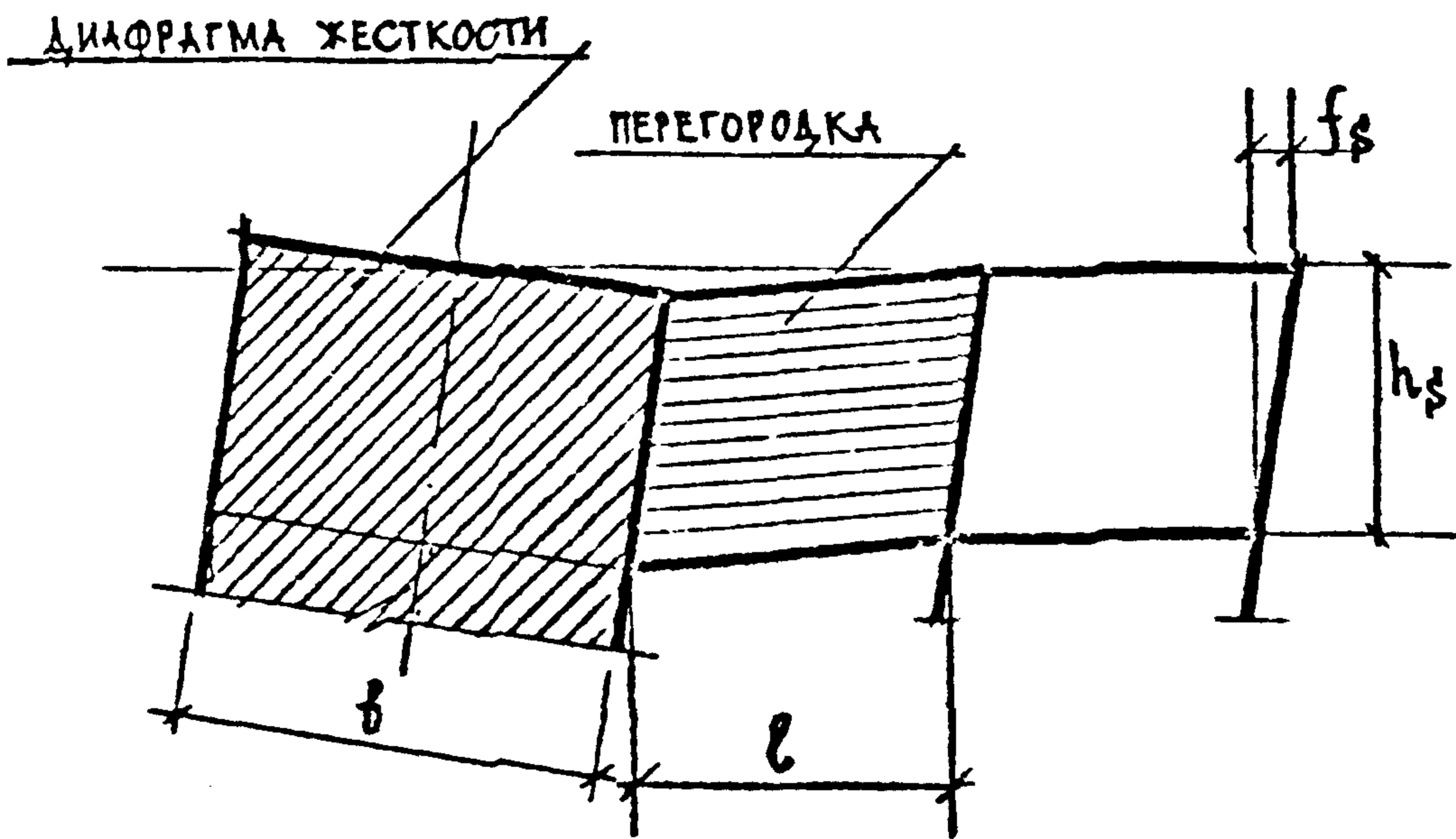
РИС. 10. СХЕМА ДЕФОРМАЦИЙ ВЕРХНЕГО ЭТАЖА ЗДАНИЯ.
