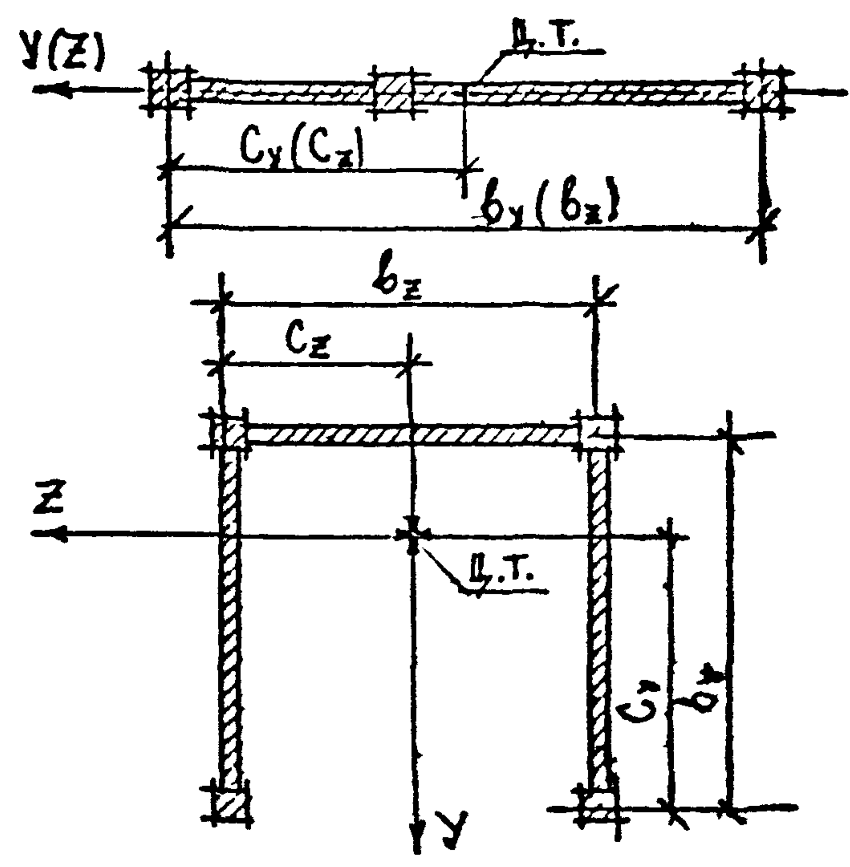
Рис. 9. К РАСЧЕТУ МНОГОКОЛОННЫХ ДИАФРАГМ Вх 32826 и 20
