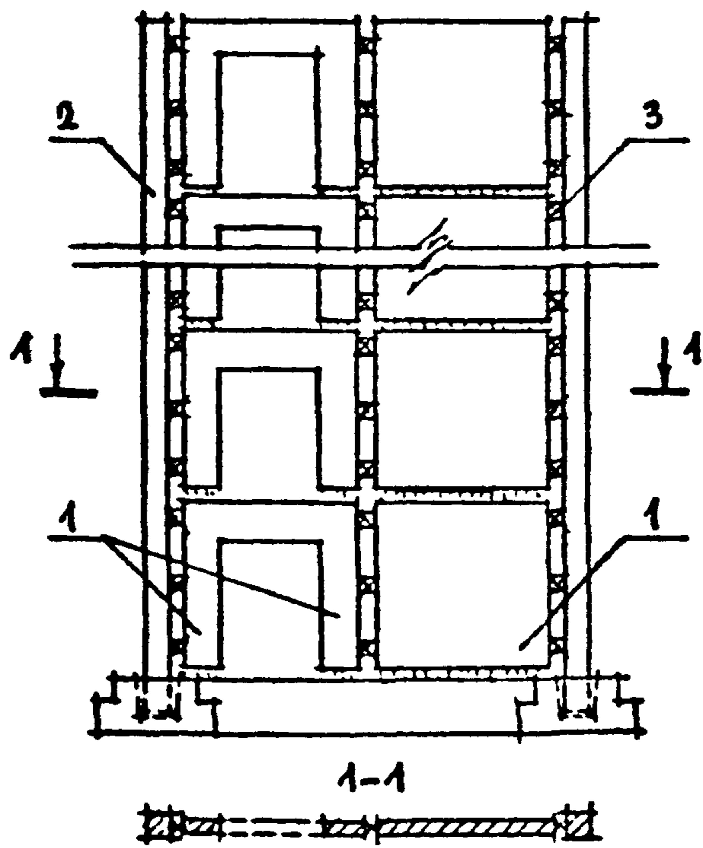
Рис. 1. Обобщенная конструктивная схема диафрагмы. 1 - стенки жесткости; 2 - диафрагменные колонны каркаса; 3 - закладные изделия
