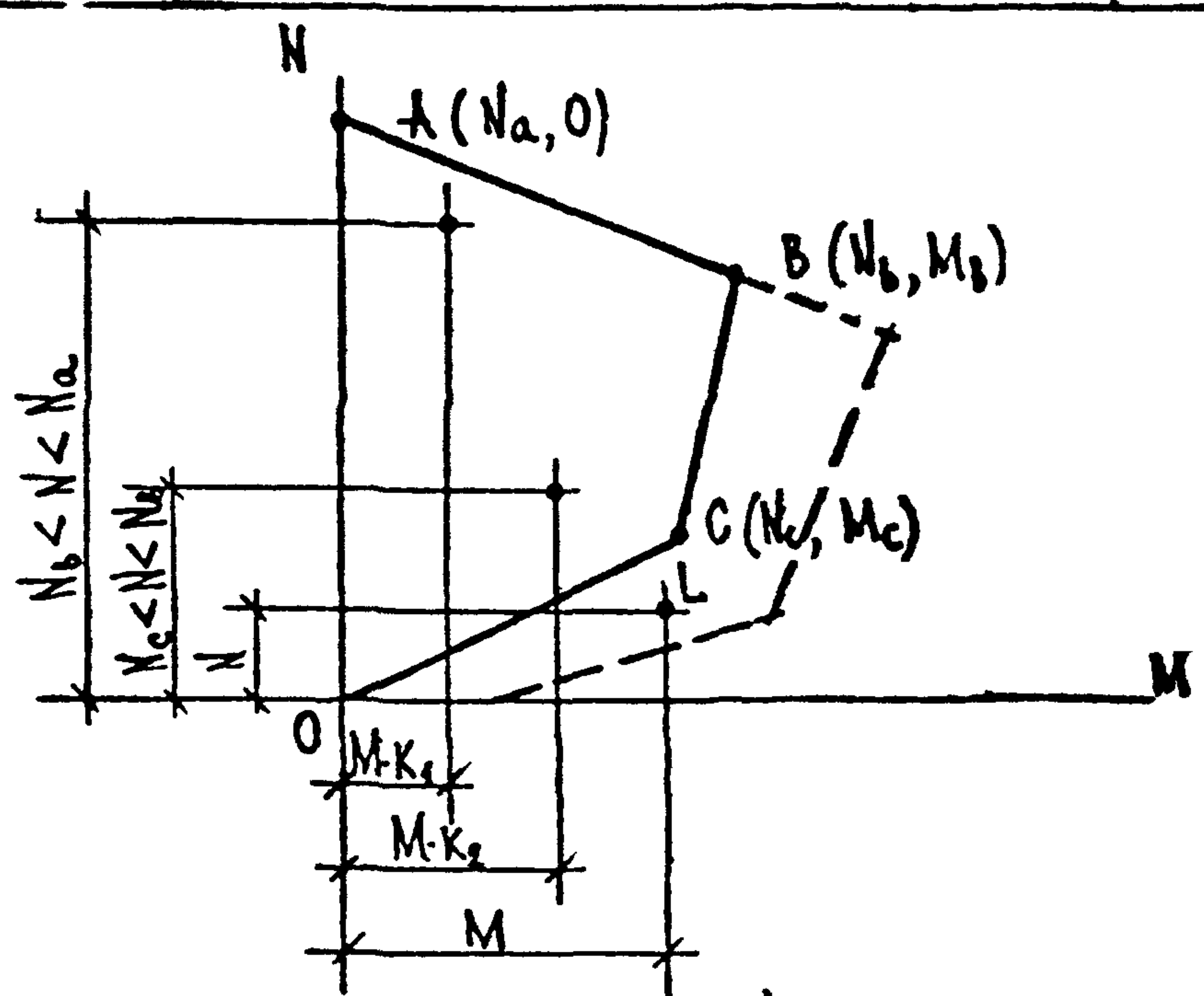
Рис. 8. ГРАФИК НЕСУЩЕЙ СПОСОБНОСТИ ВНЕЦЕНТРЕННО СЖАТОЙ ДИАФРАГМЫ.
