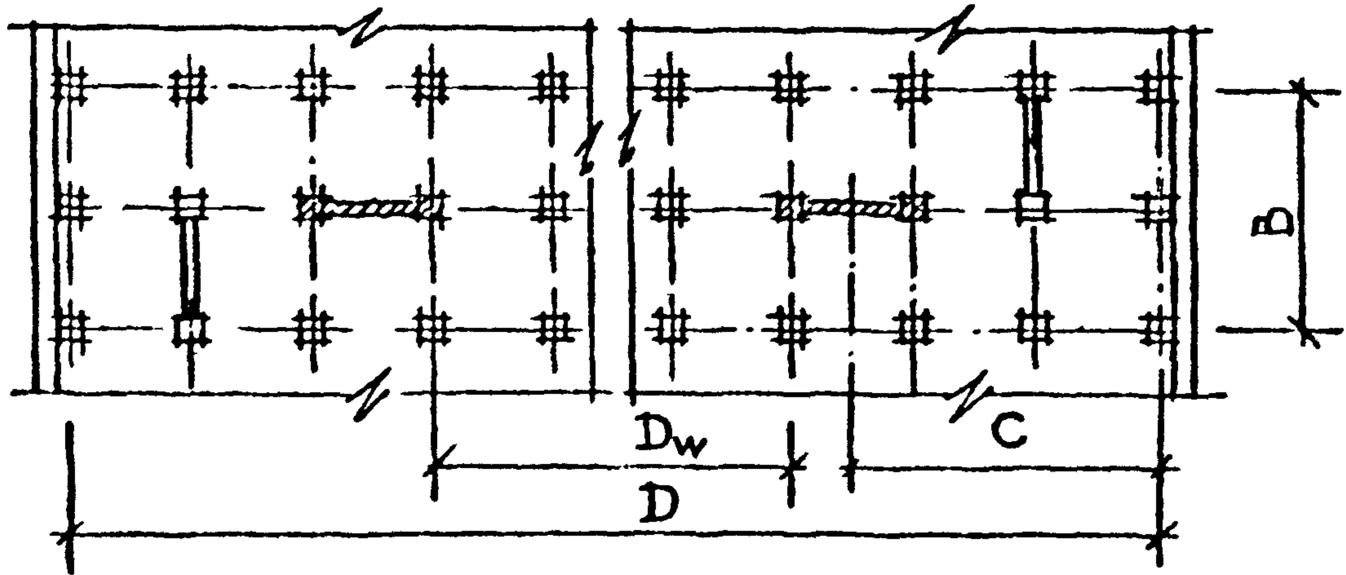
Рис. 16. ПРЕДЕЛЬНЫЕ ГАБАРИТЫ ЗДАНИЯ И РАССТОЯНИЯ МЕЖДУ ДИАФРАГМАМИ.
