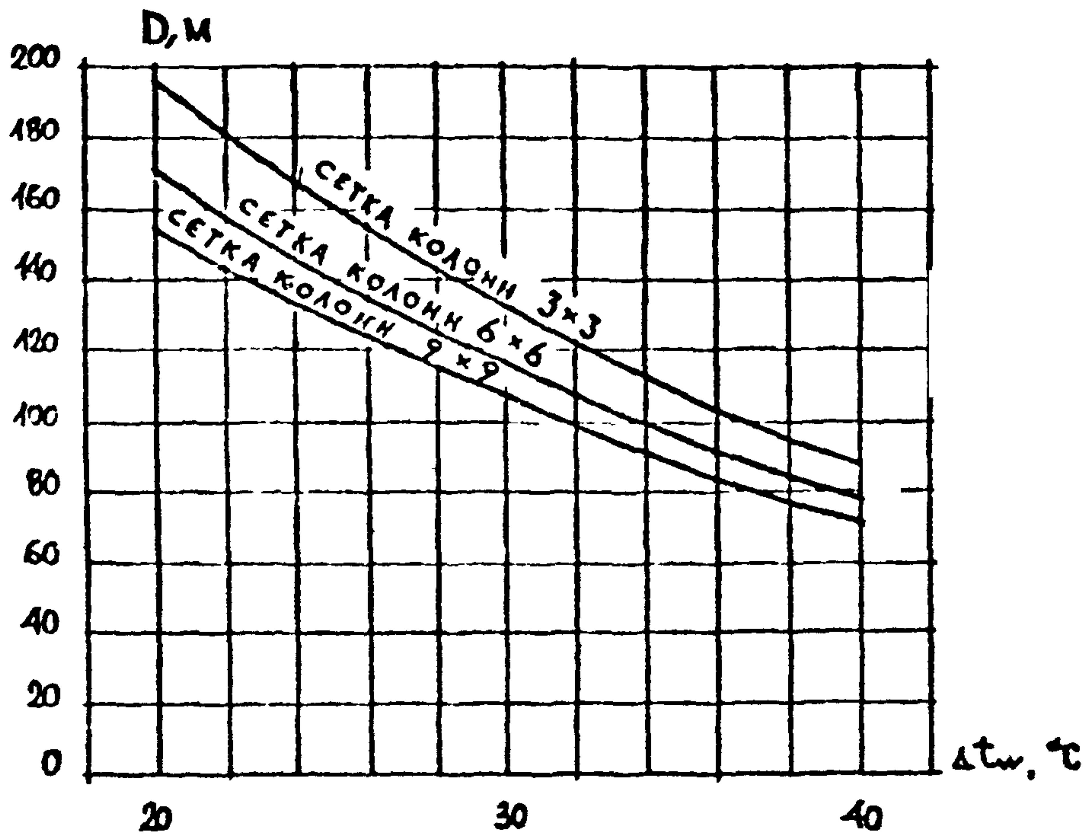
Рис. 17. ДОПУСТИМЫЕ ГАБАРИТЫ ЗДАНИЯ ПРИ РАЗЛИЧНОЙ СЕТКЕ КОЛОНН.
