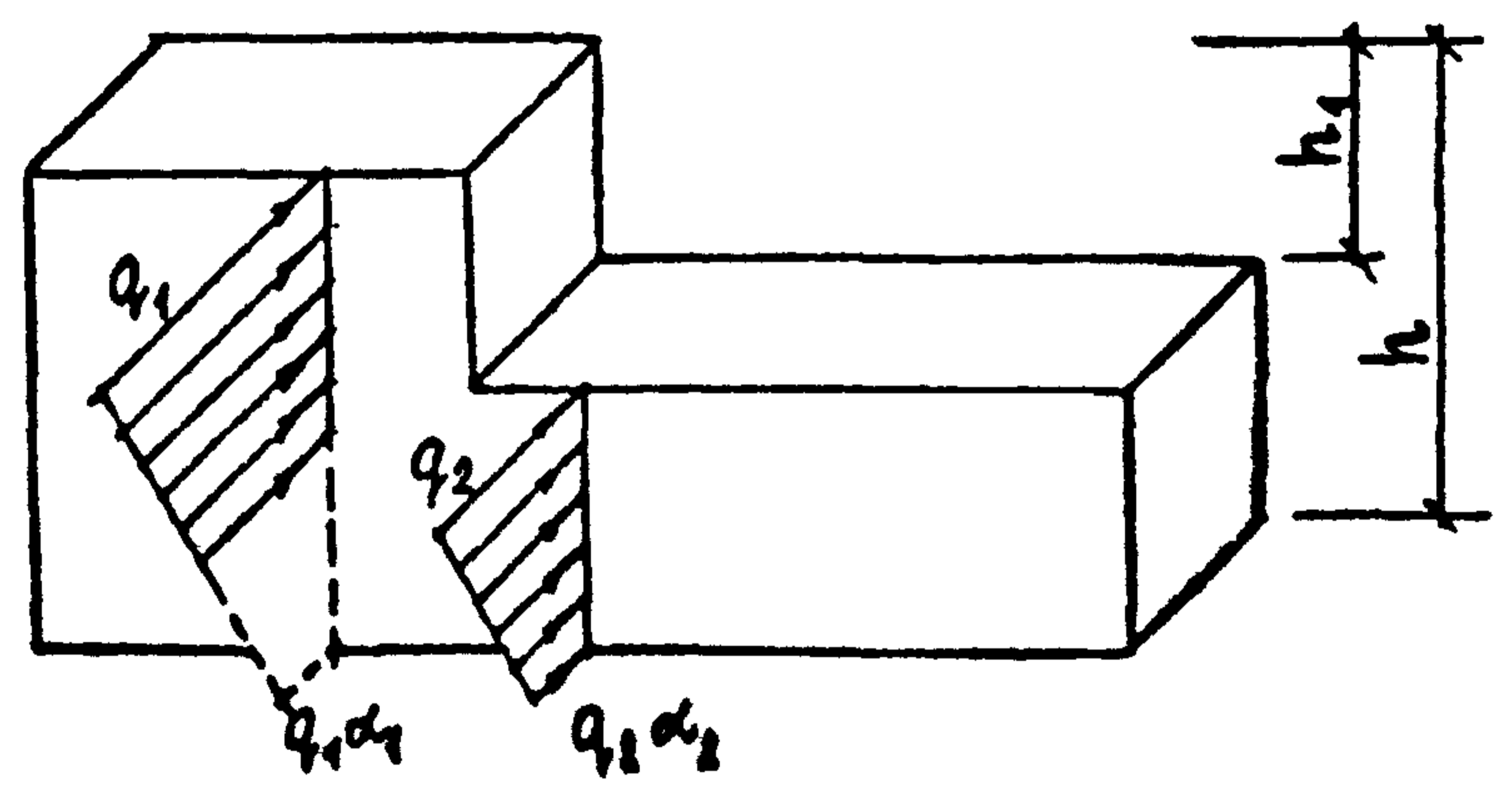
РИС. 6. СХЕМА ЗДАНИЯ ПЕРЕМЕННОЙ ВЫСОТЫ. Вх. 32826. Л 13
