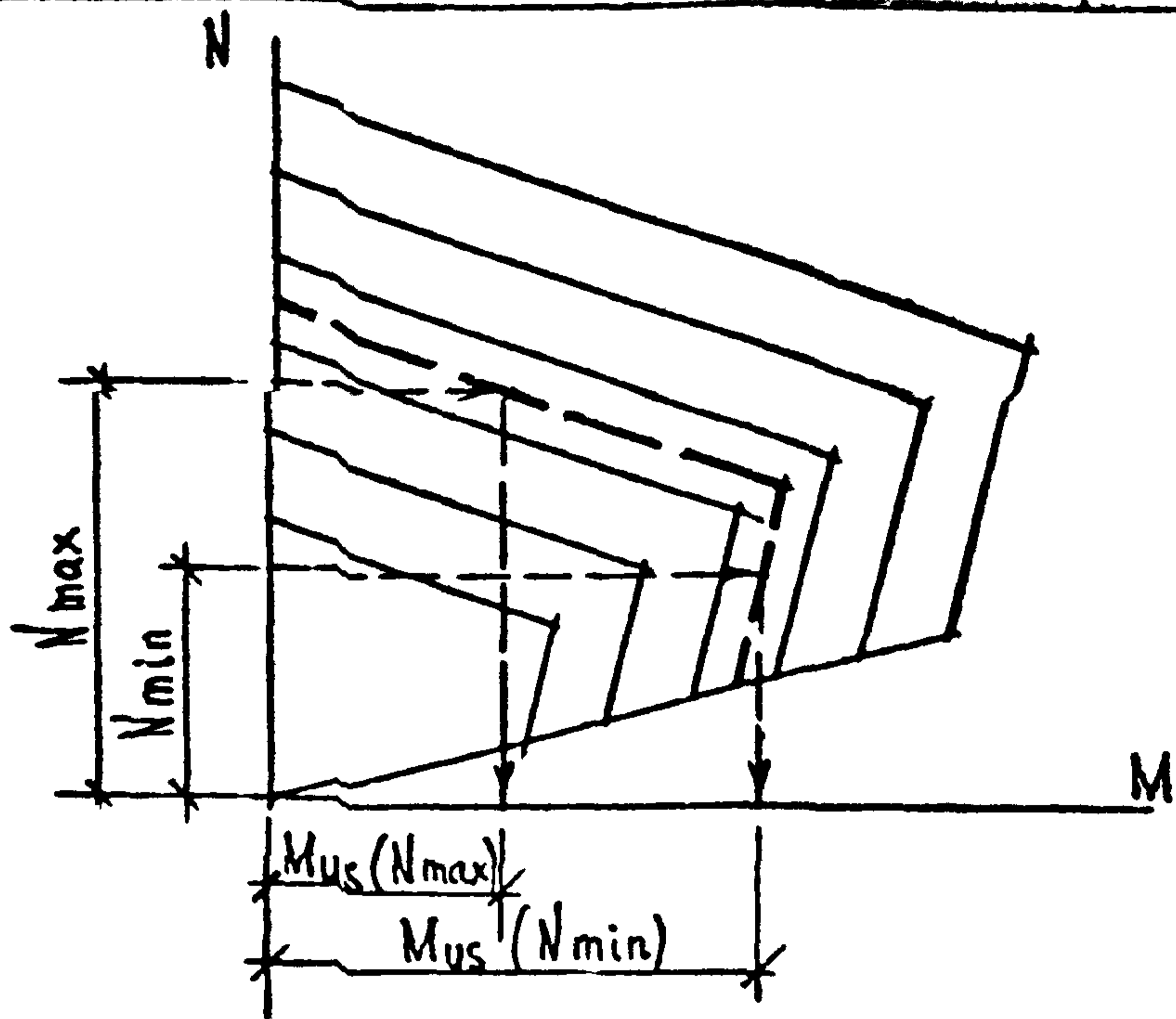
Рис. 11. ОПРЕДЕЛЕНИЕ ПРЕДЕЛЬНО ДОПУСТИМЫХ МОМЕНТОВ ДИАФРАГМ.
