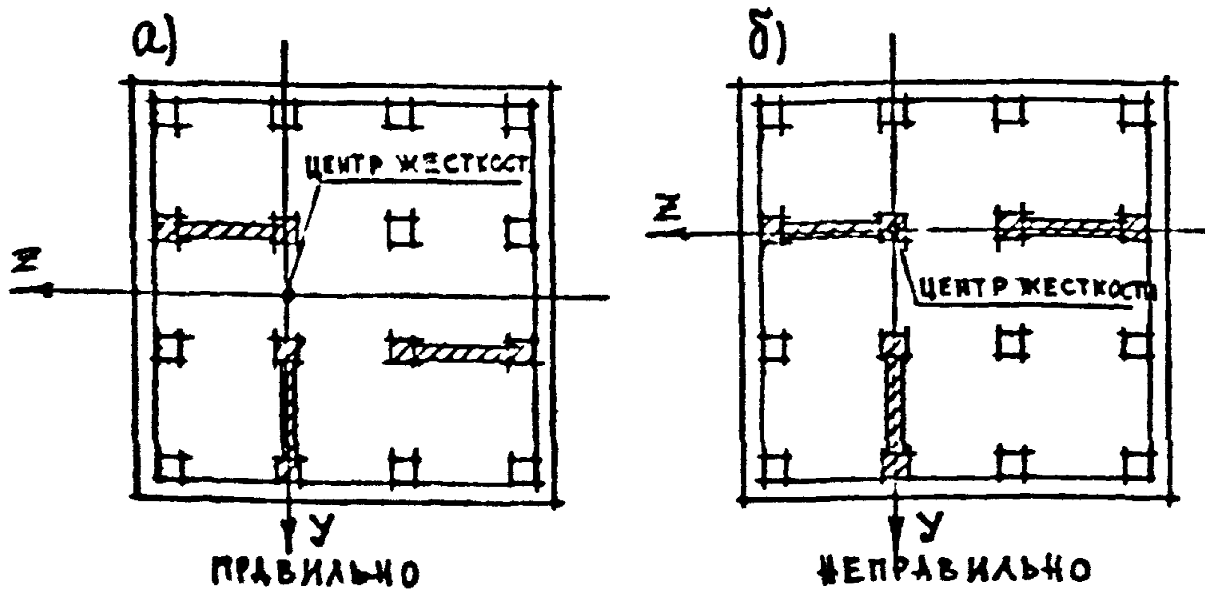
Рис. 2. Примеры правильной (а) и неправильной (б) компоновки конструктивной схемы здания Вх. 32826 л 7
