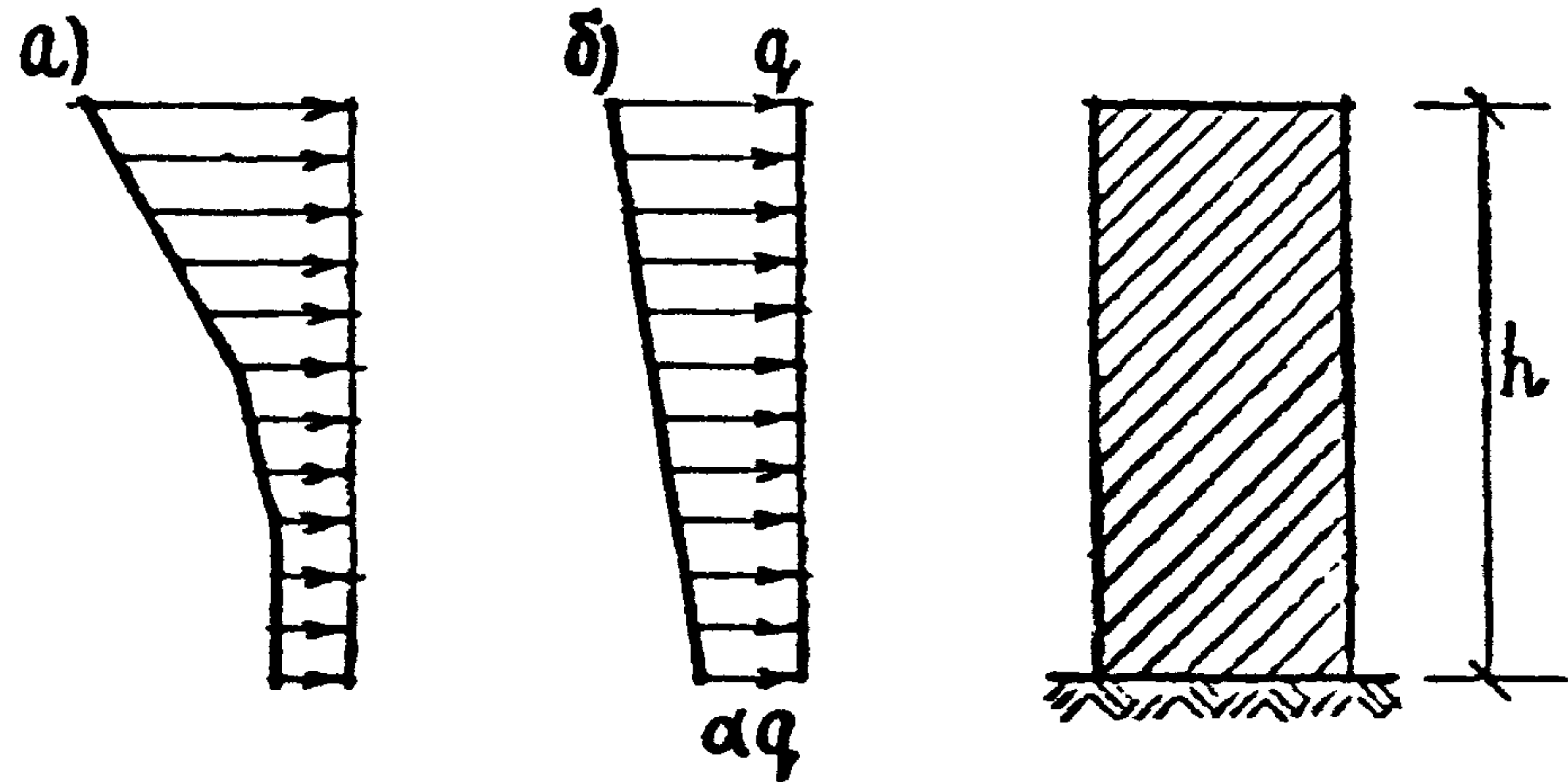
РИС. 4. ДЕЙСТВИТЕЛЬНАЯ (α) И РАСЧЕТНАЯ (δ) ЭПЮРЫ ВЕТРОВЫХ НАГРУЗОК.
